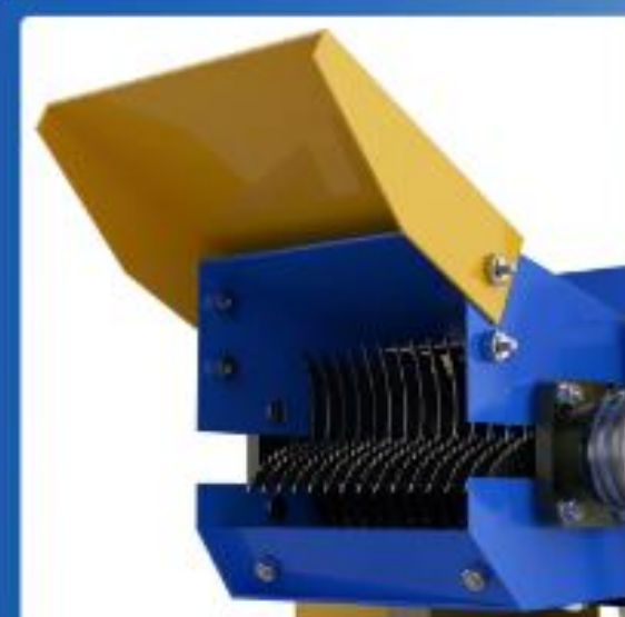
Outlet baffle
